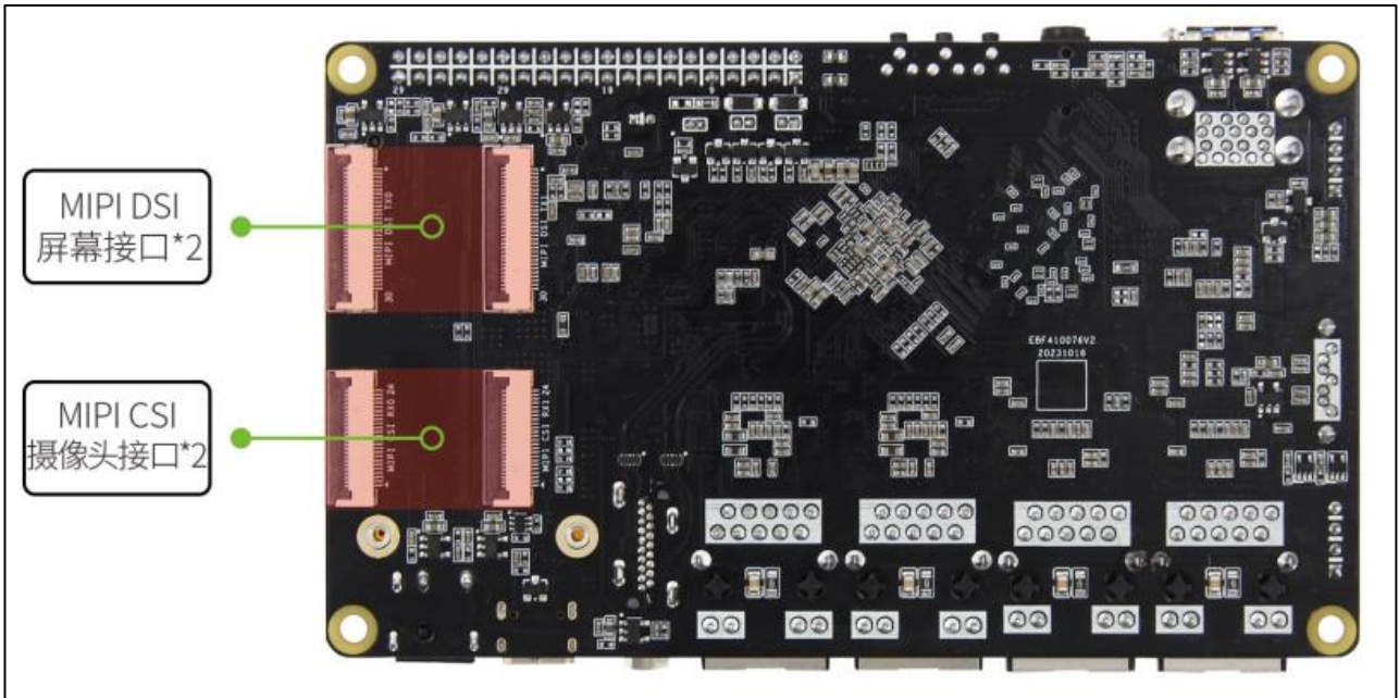
图 3.2.1-3 鲁班猫 2N 背面视图
