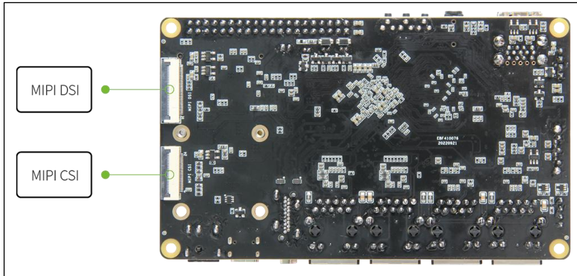
图 3.2.1-6 鲁班猫 2N-V2 背面视图
