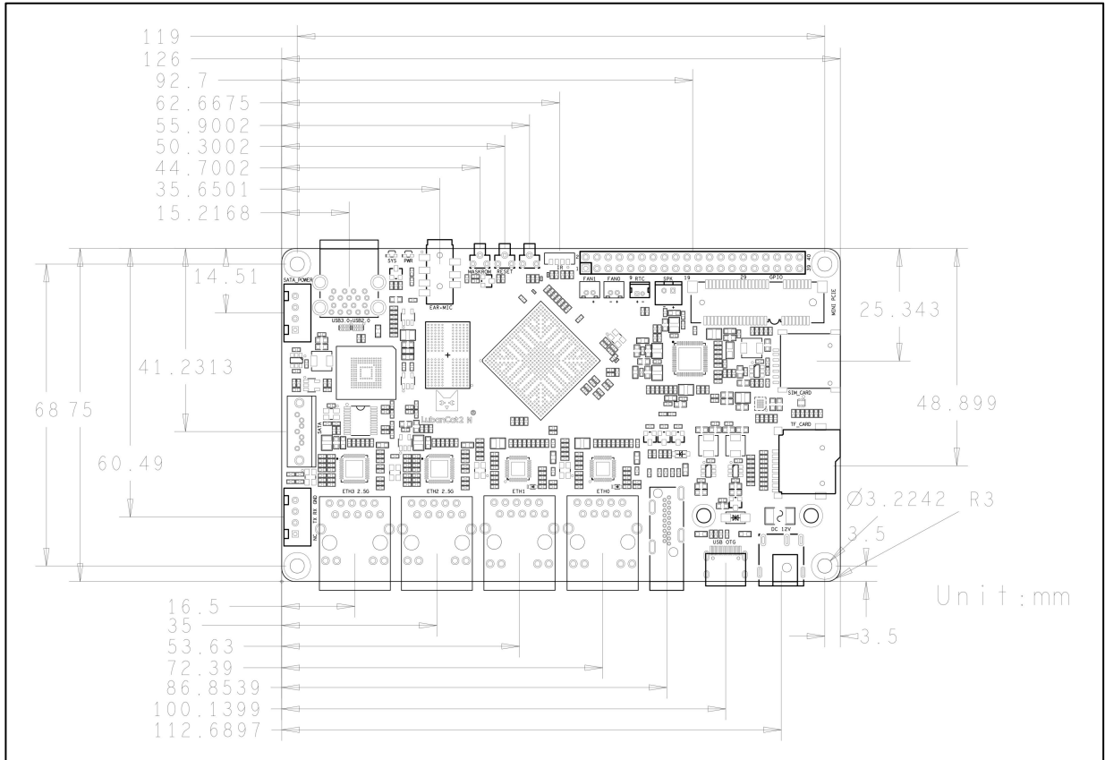
图 3.2.2-2 鲁班猫 2N-V2 机械尺寸图
